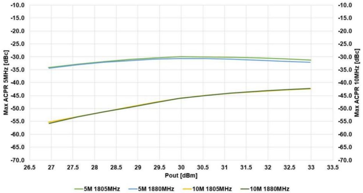
WCDMA, ACPR_5MHz, ACPR_10MHz vs Pout
