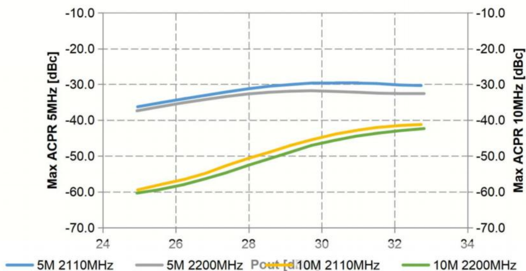
WCDMA, ACPR_5MHz, ACPR_10MHz vs Pout
