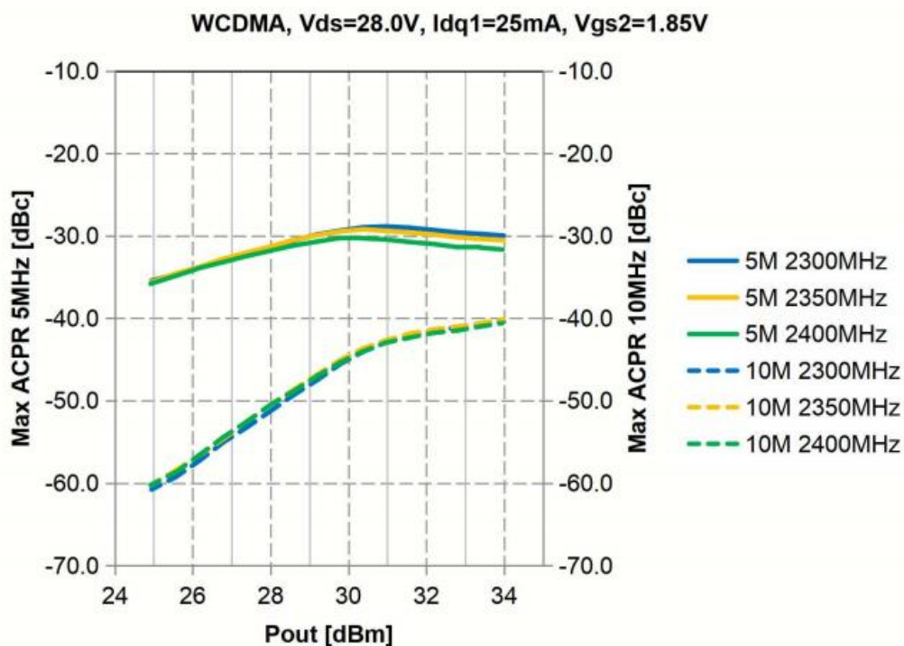
WCDMA, ACPR_5MHz, ACPR_10MHz vs Pout
