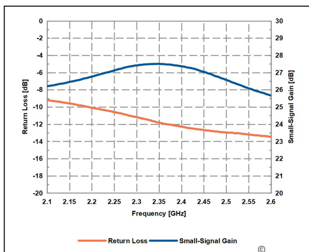
S-Parameter
