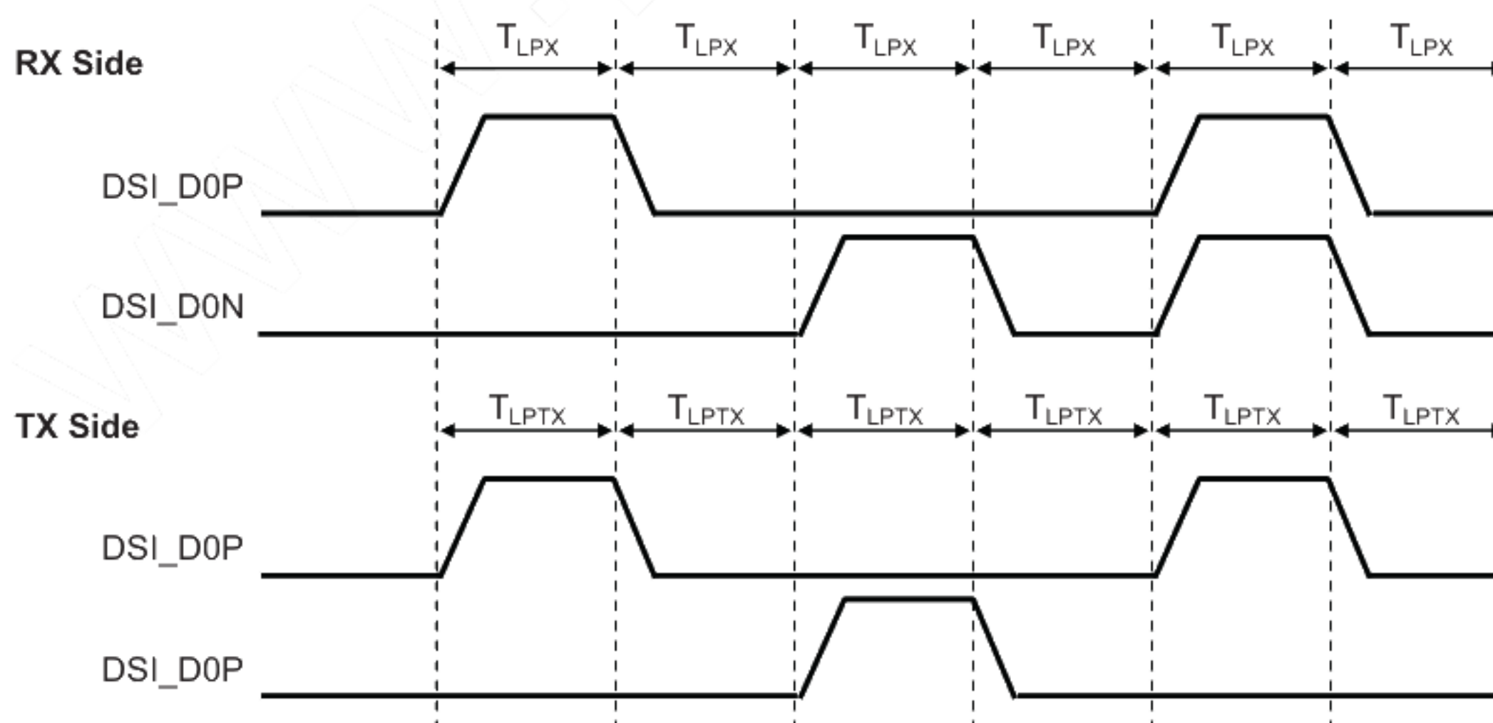
Fig.E DSI LP Mode
