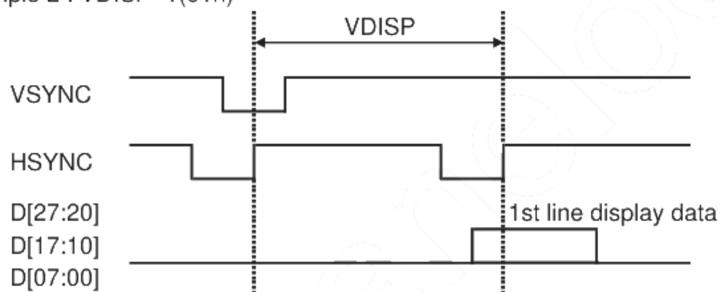
Example 2 : VDISP=1(01h)
