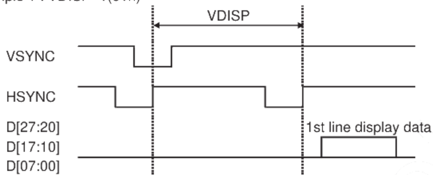
Example 1 : VDISP=1(01h)
