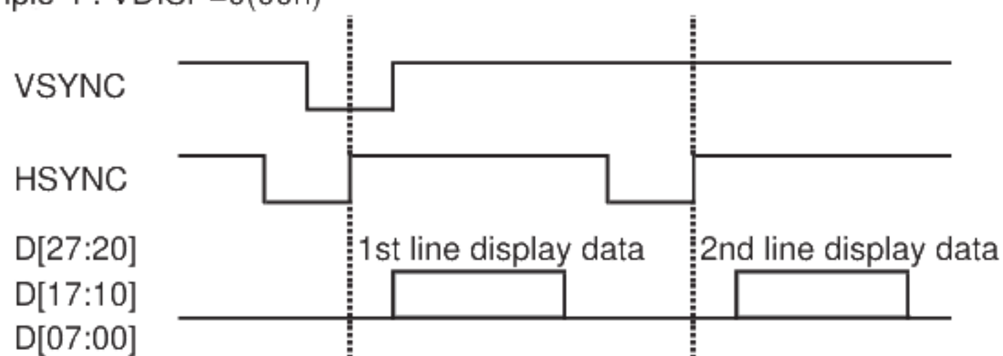
Example 4 : VDISP=0(00h)
