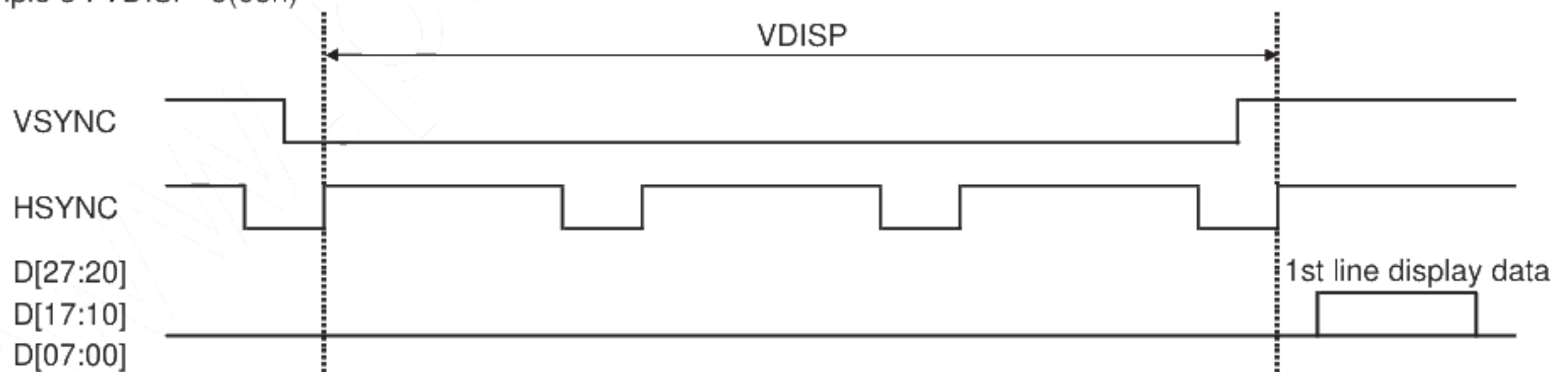
Example 3 : VDISP=3(03h)
