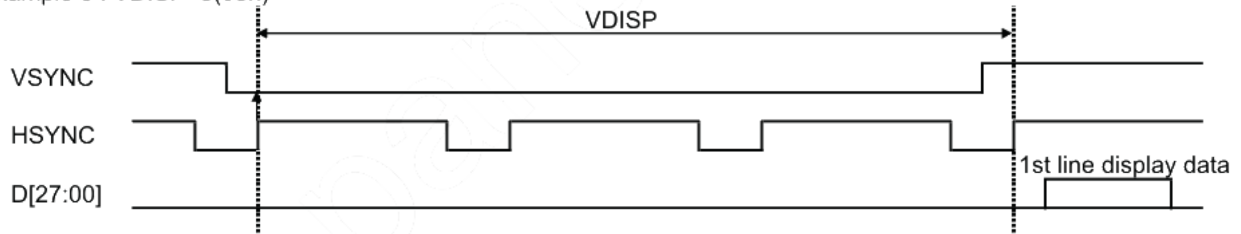
Example 3 : VDISP=3(03h)
