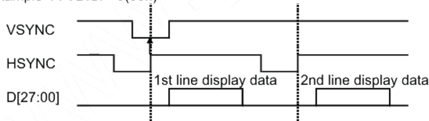
Example 4 : VDISP=0(00h)
