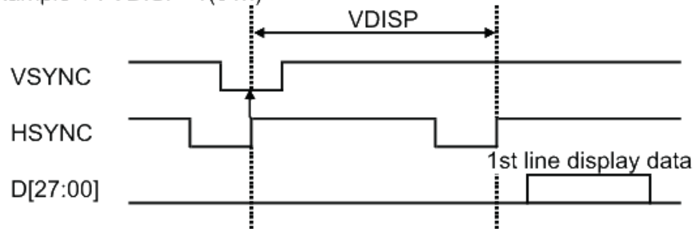
Example 1 : VDISP=1(01h)
