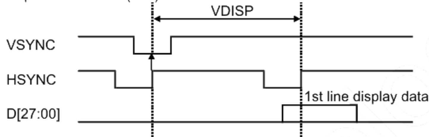
Example 2 : VDISP=1(01h)
