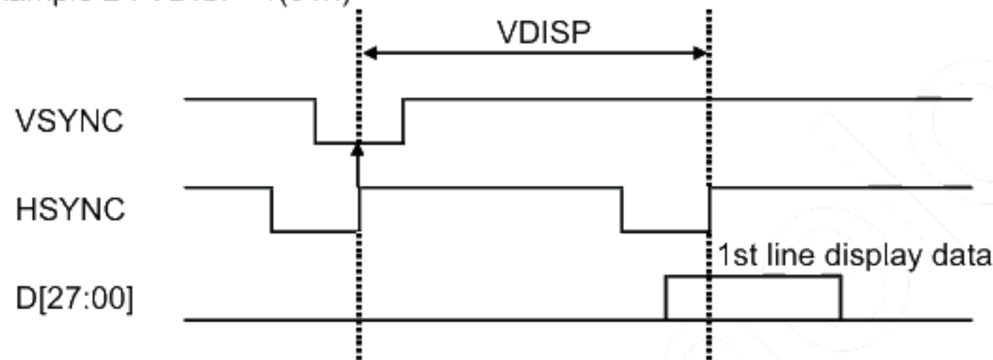
Example 2 : VDISP=1(01h)
