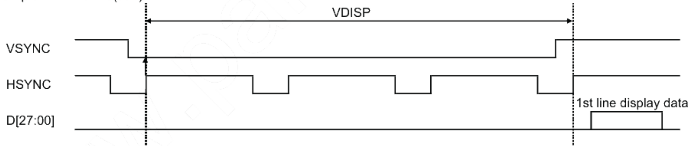
Example 3 : VDISP=3(03h)
