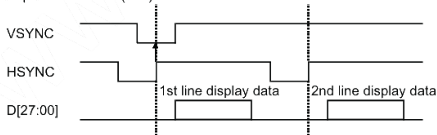
Example 4 : VDISP=0(00h)
