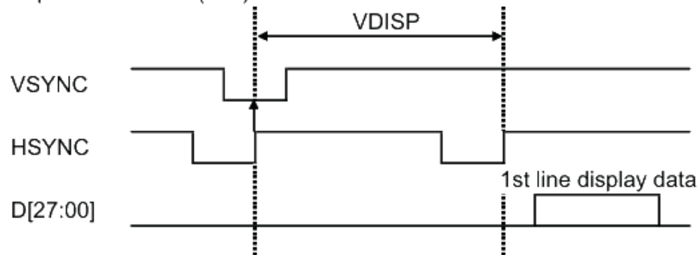
Example 1 : VDISP=1(01h)
