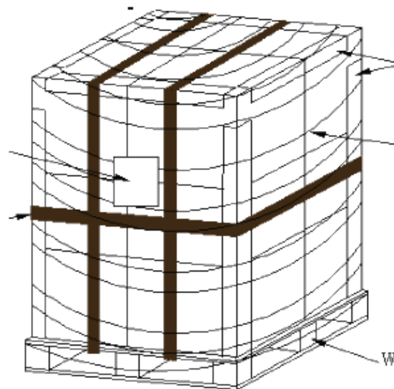
單層 pallet 打棧示意圖
