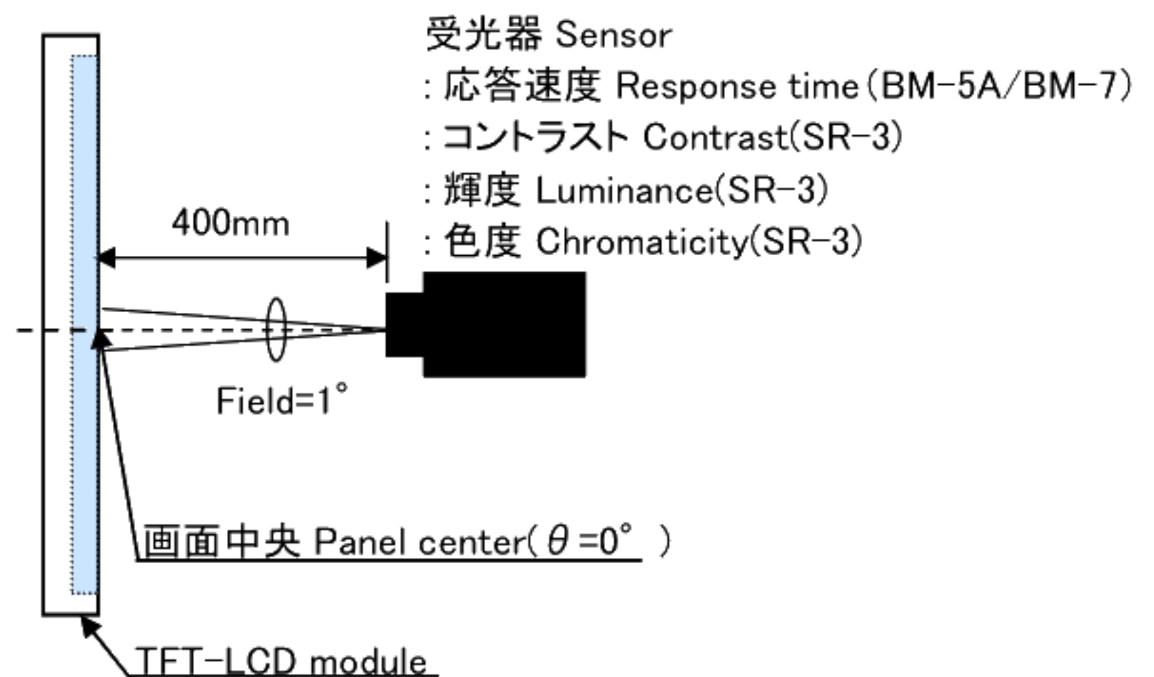
図3-2 コントラスト/輝度/応答速度/色度特性測定方法
