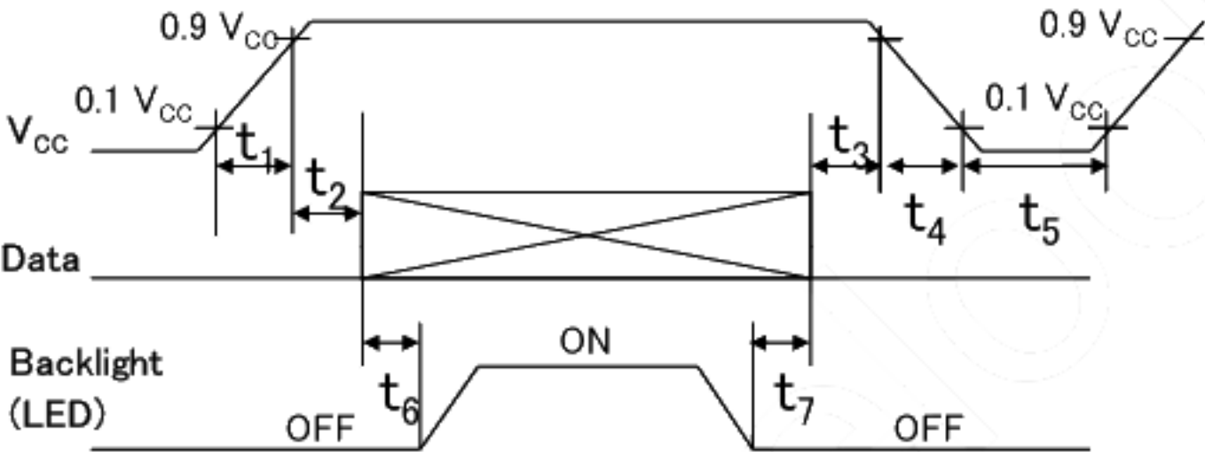
【Note1】 入力電圧シーケンス Vcc turn-on/off conditions
