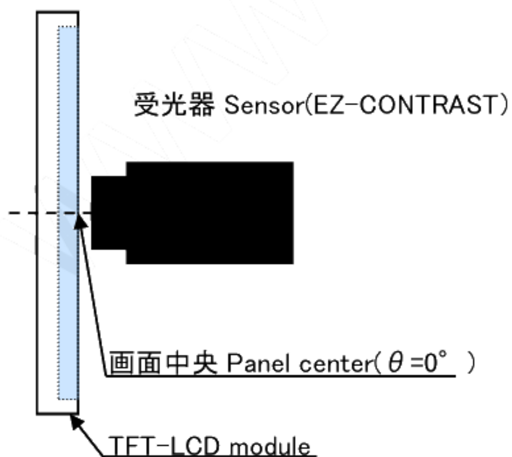
図3-1 視野角特性測定方法
