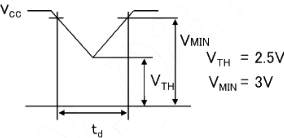
瞬時電圧降下 Vcc-dip conditions
