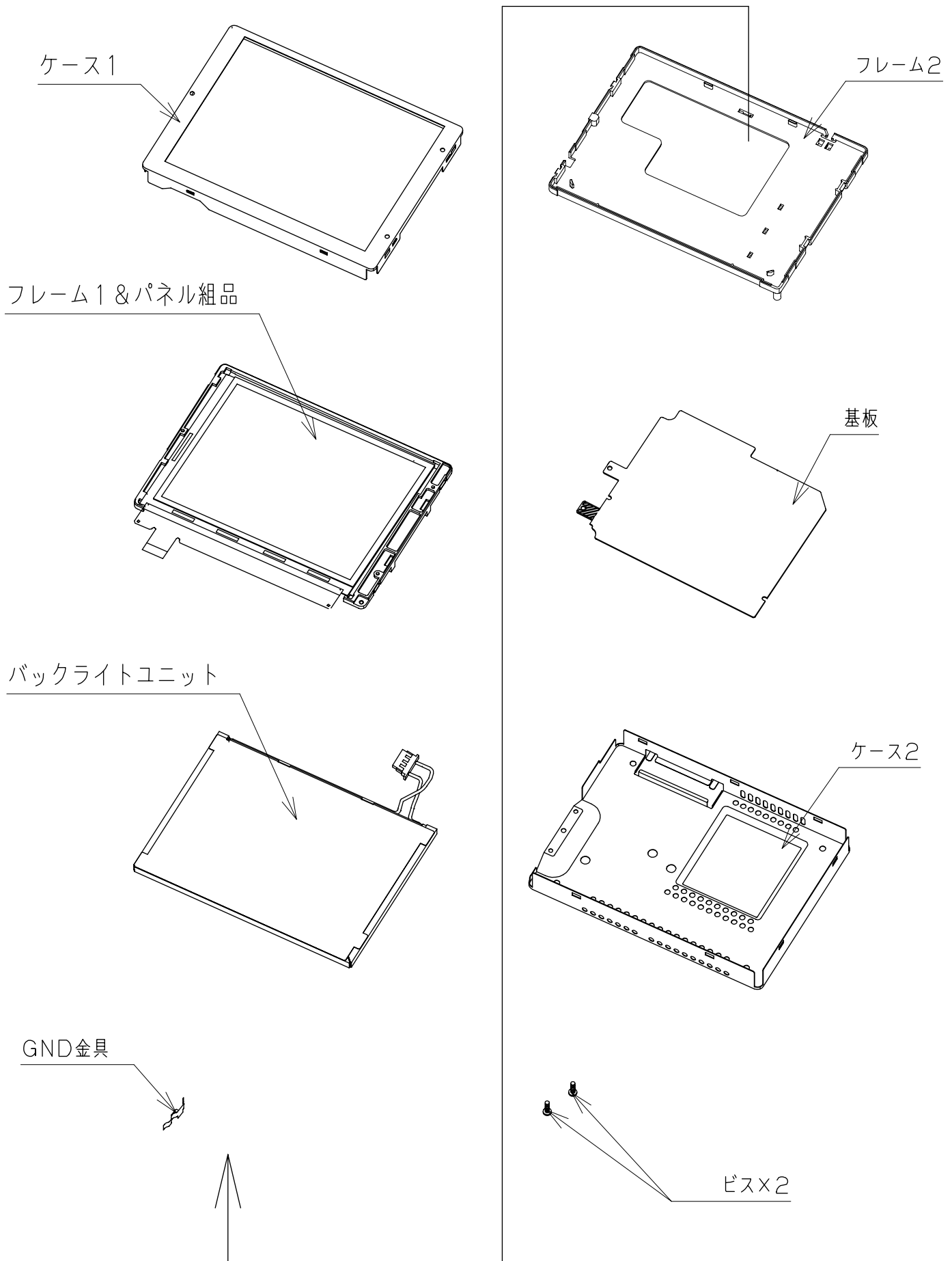
図2. モジュール組立て形態図
