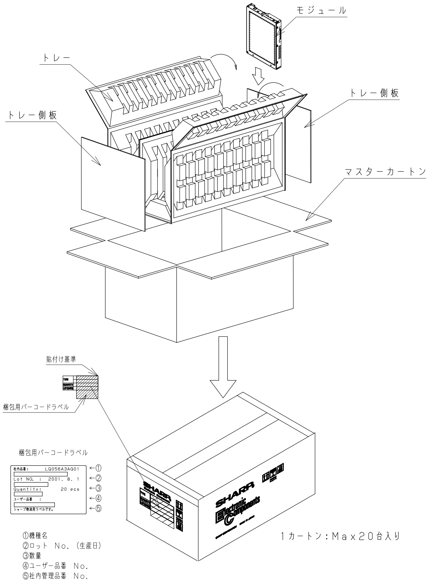
図8. 梱包形態図
