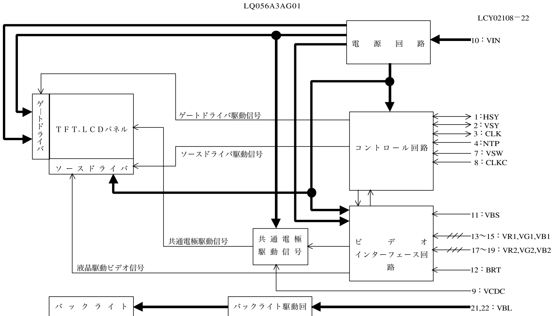
図4 モジュール回路ブロック図
