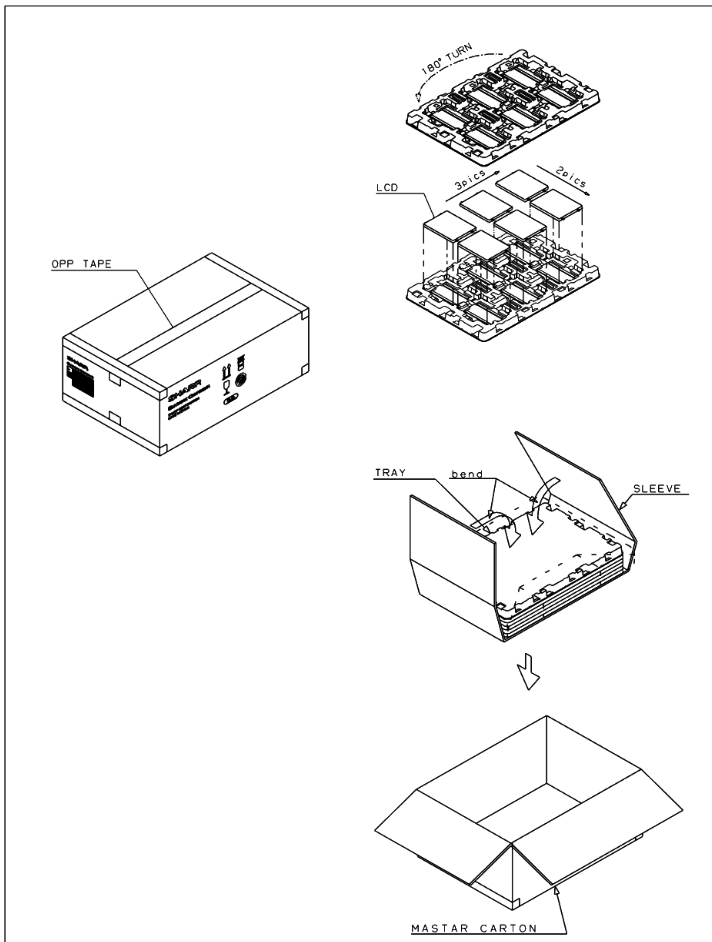
图3：包装形态图 Fig3：Packing form figure
