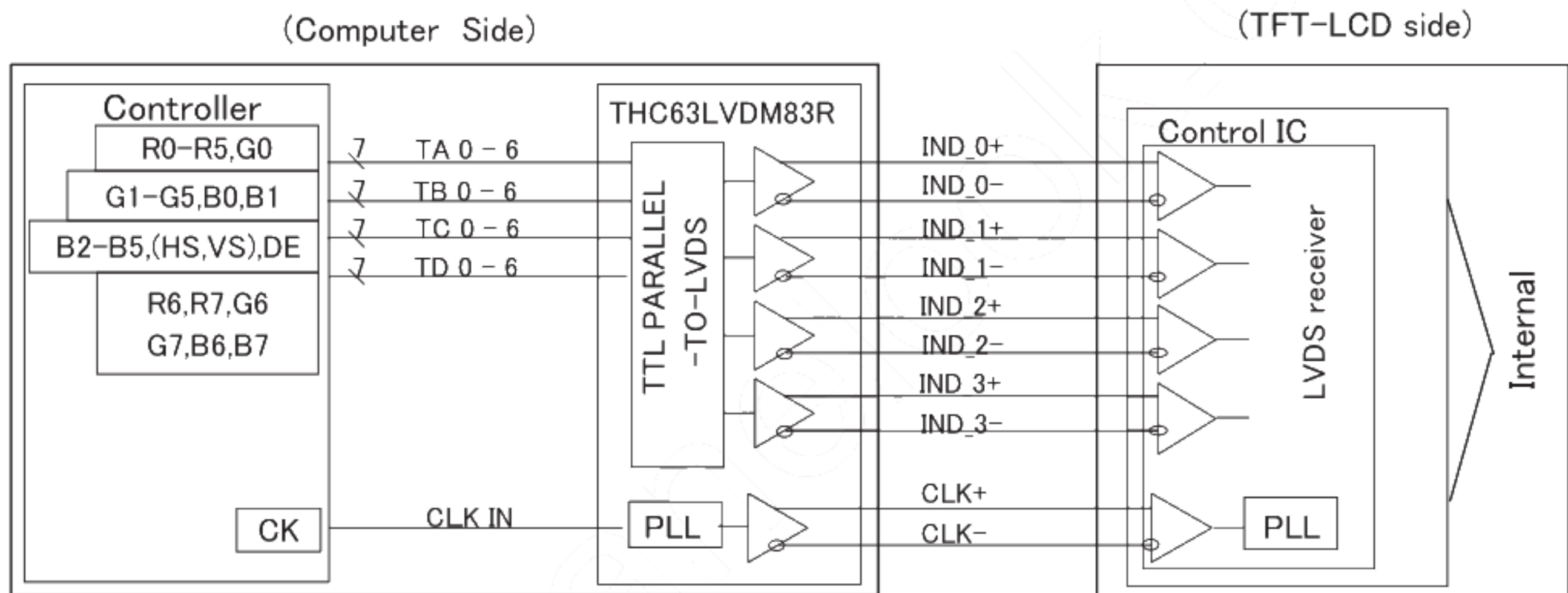
4-3. LVDSインターフェイスブロック図 LVDS interface block diagram
