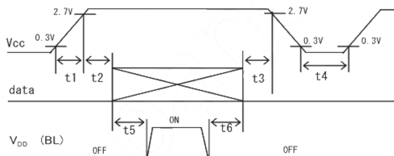
【Note6-1】 入力電圧シーケンス V_{CC} turn-on/off conditions
