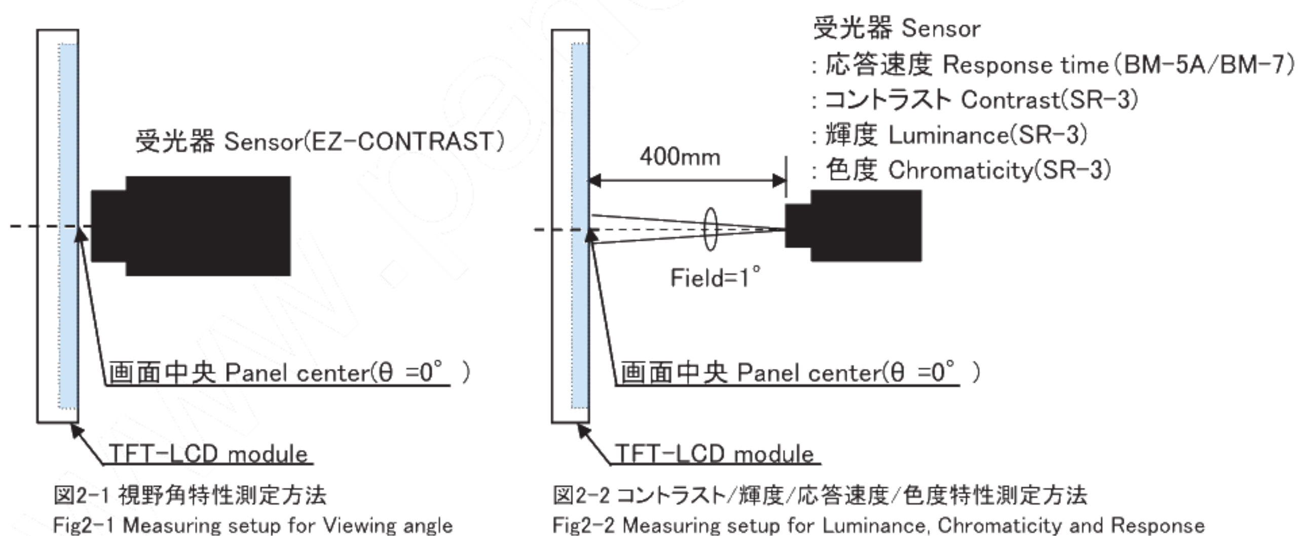
図2 光学的特性測定方法
