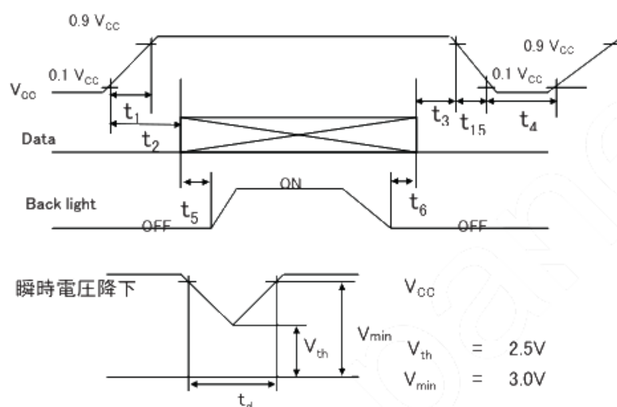
【Note6-1】 入力電圧シーケンス
