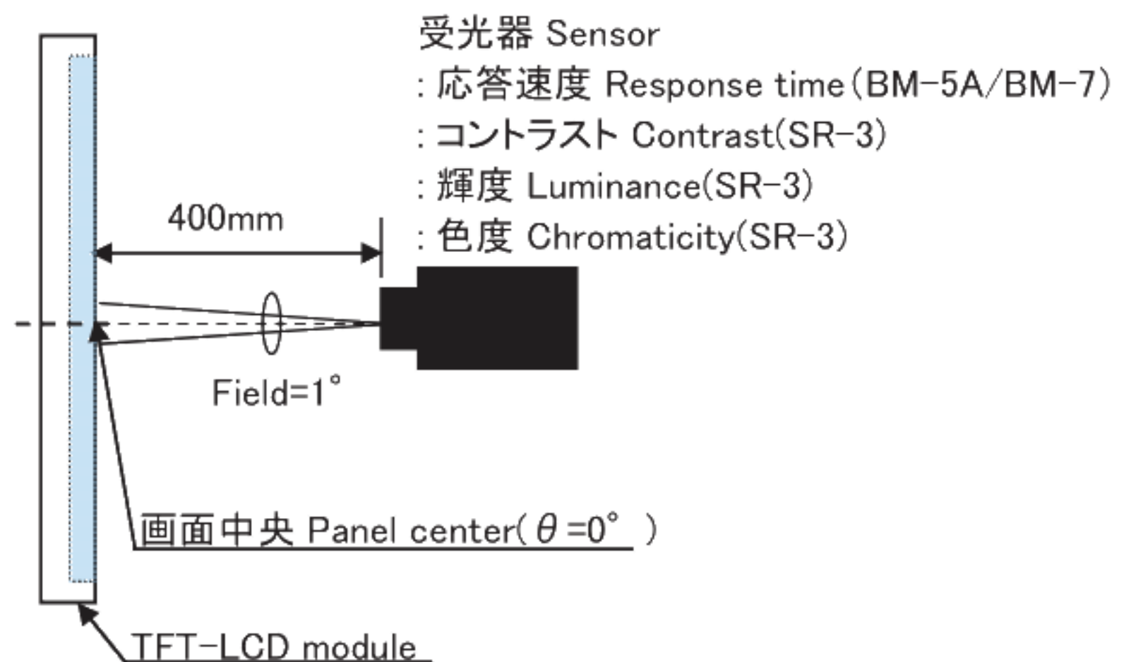
図2-2 コントラスト/輝度/応答速度/色度特性測定方法 Fig2-2 Measuring setup for Luminance, Chromaticity and Response time
