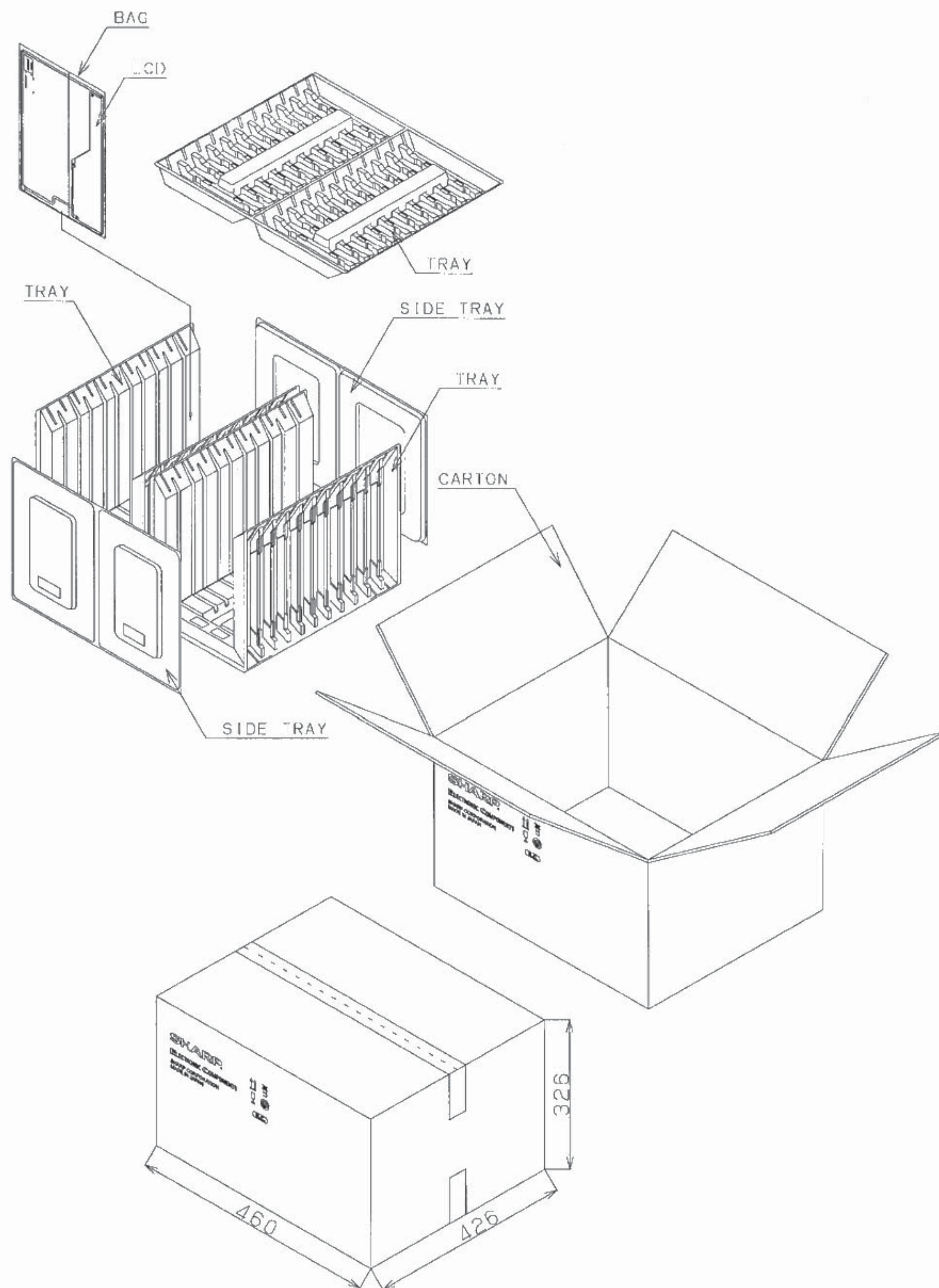
図3. 包装形態図
