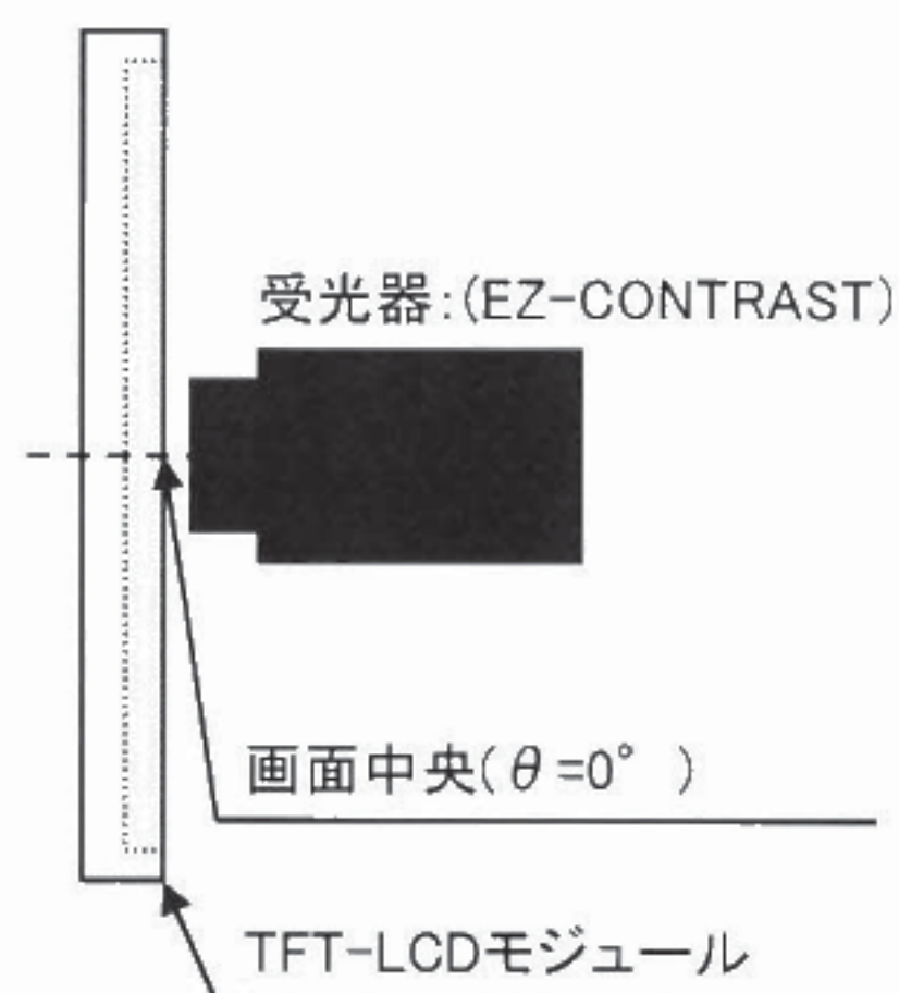
図2-1 視野角特性測定方法
