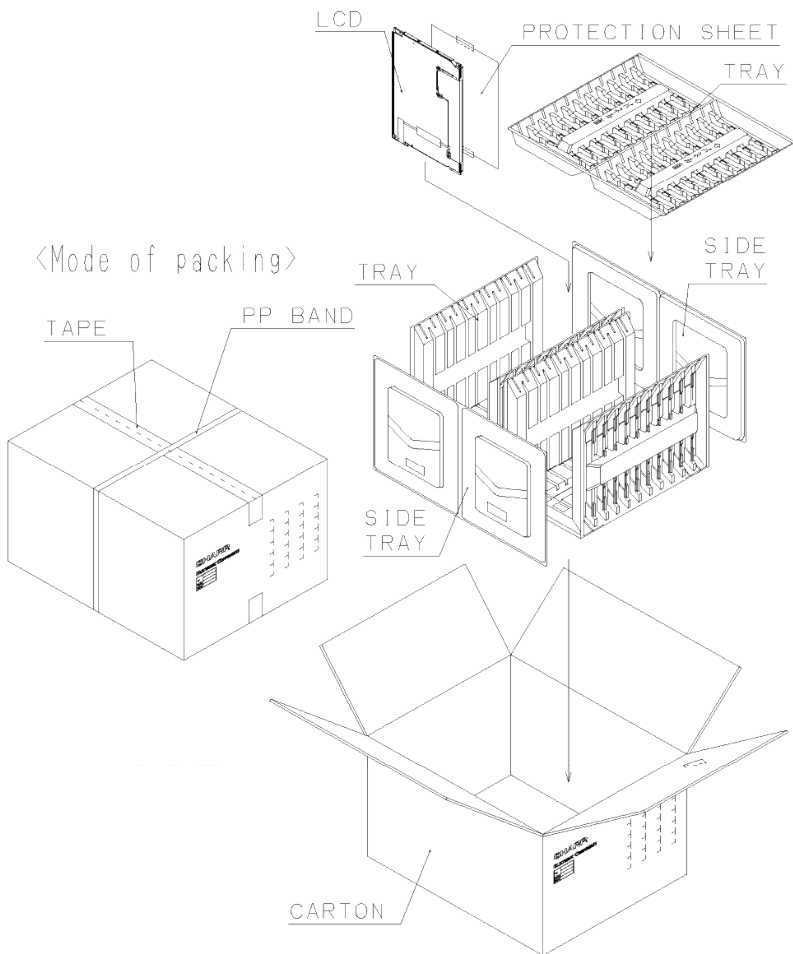
图3. 包装形态图
