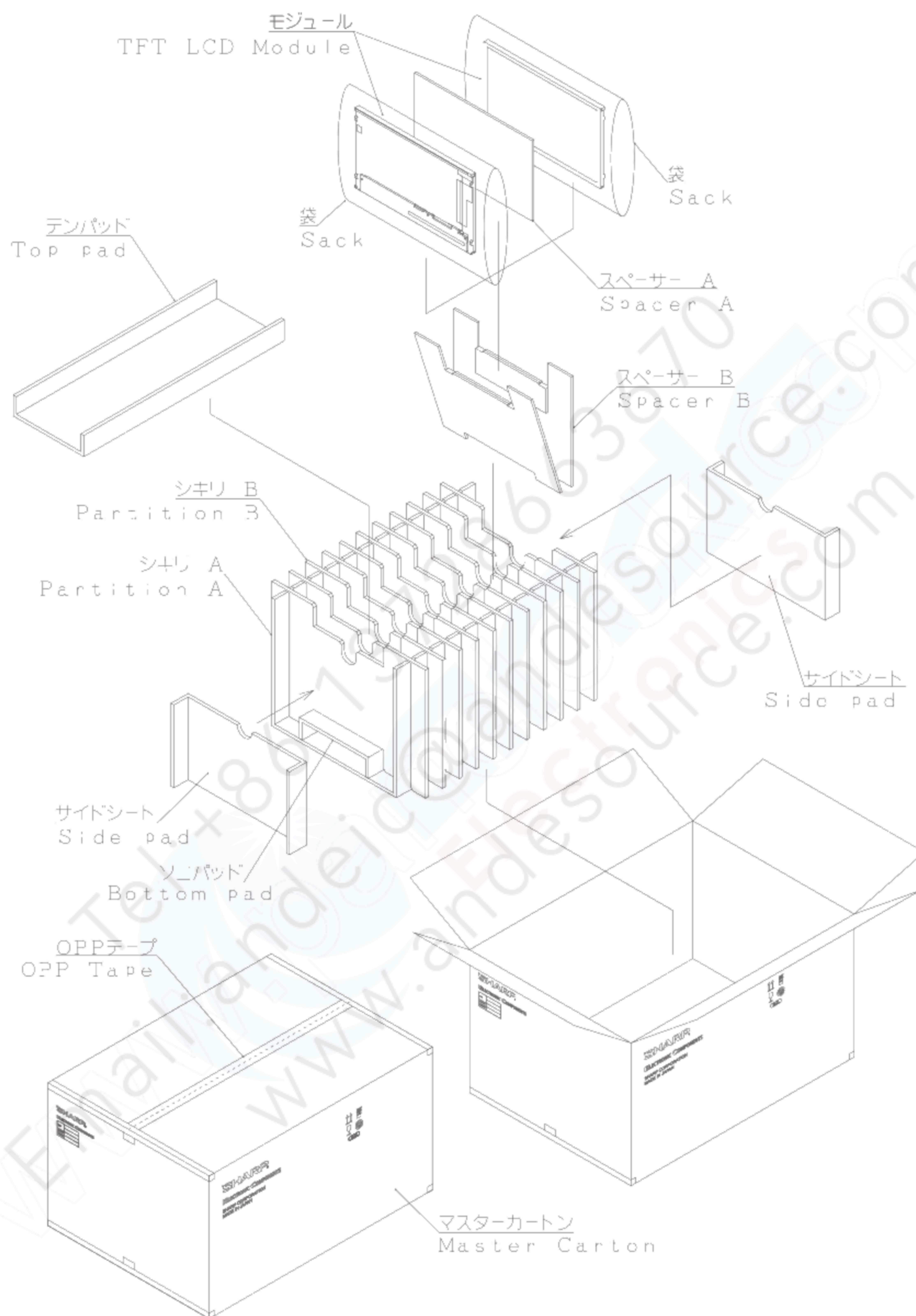
図3 包装形態図
