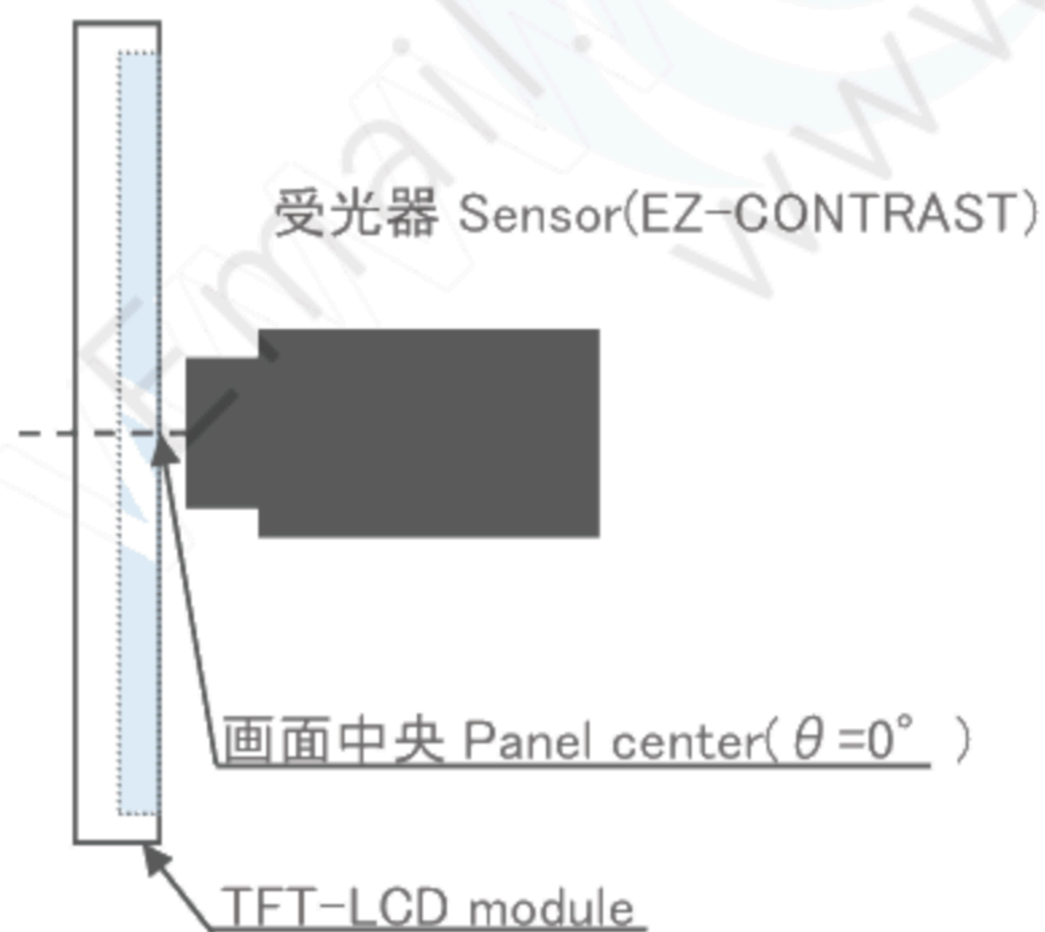
図2-1 視野角特性測定方法
