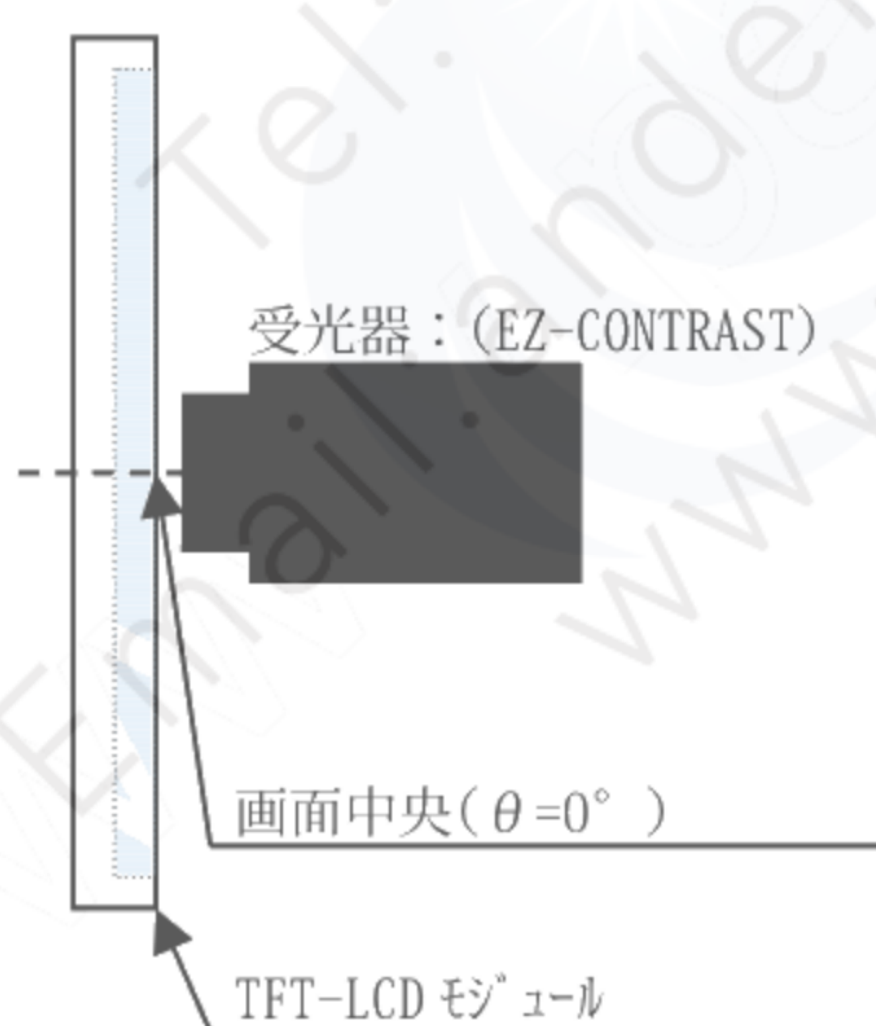
図 2-1 視野角特性測定方法
