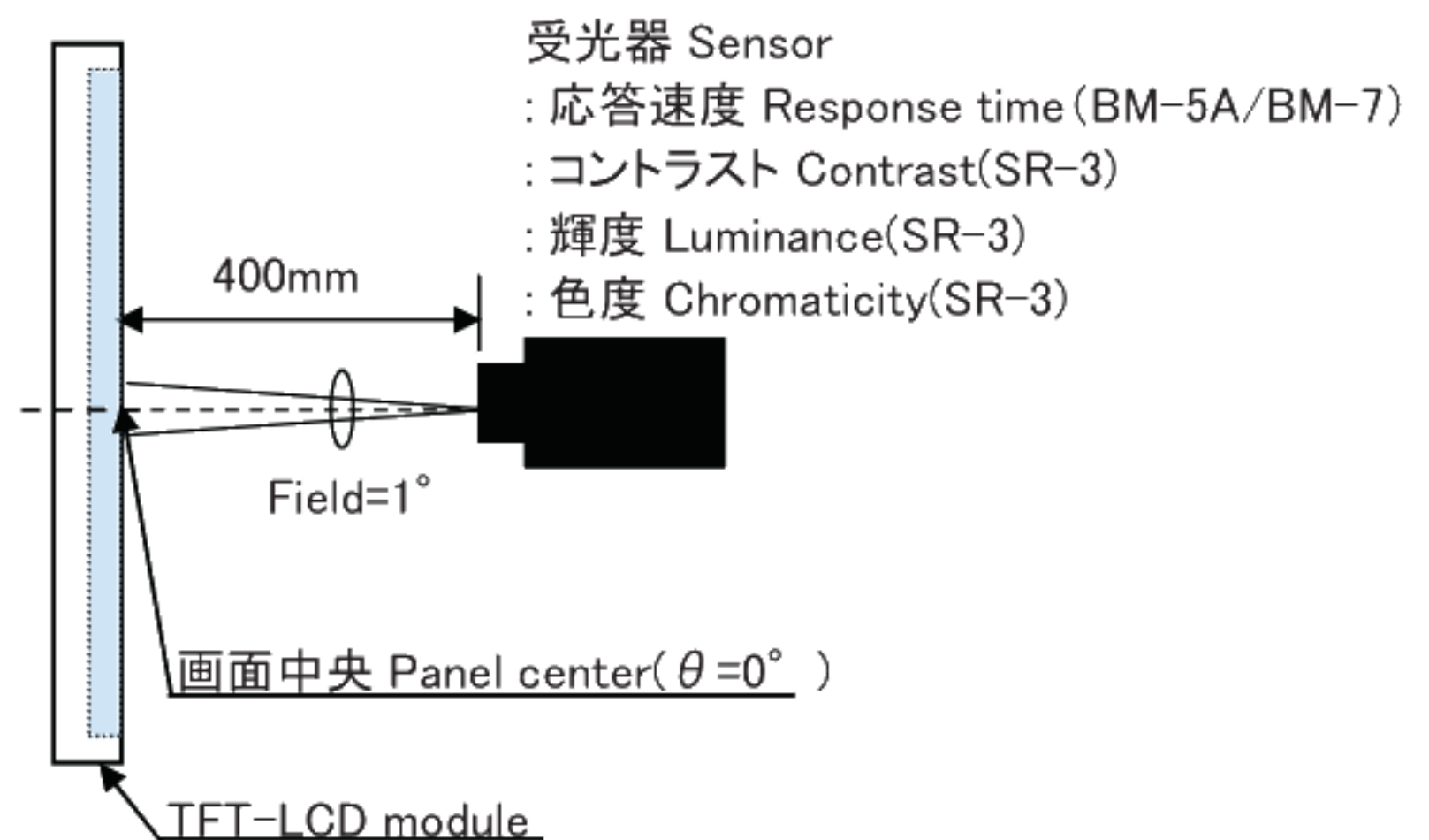
図2-2 コントラスト/輝度/応答速度/色度特性測定方法
