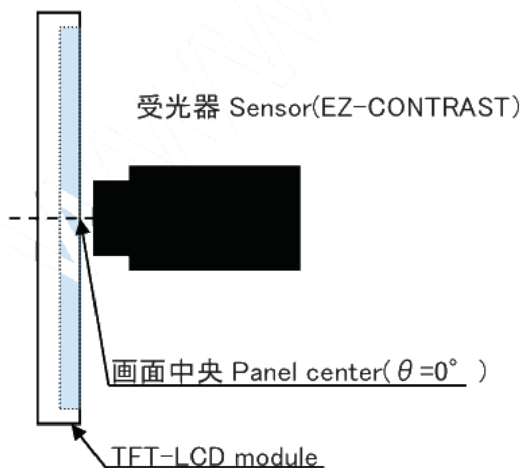
図2-1 視野角特性測定方法
