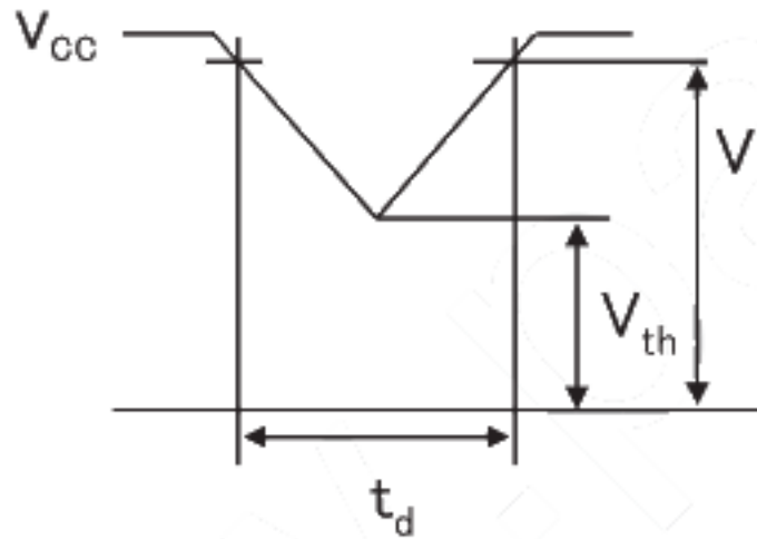
瞬時電圧降下 Vcc-dip conditions
