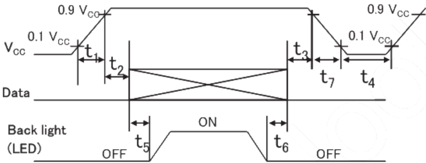
【Note1】 入力電圧シーケンス Vcc turn-on/off conditions
