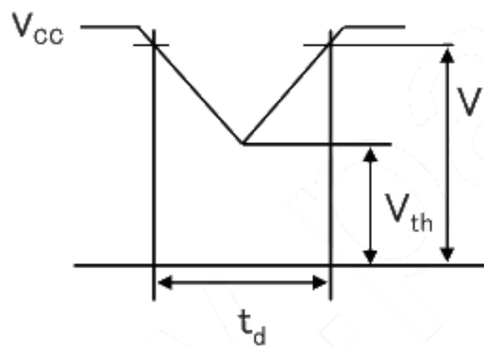
瞬時電圧降下 Vcc-dip conditions
