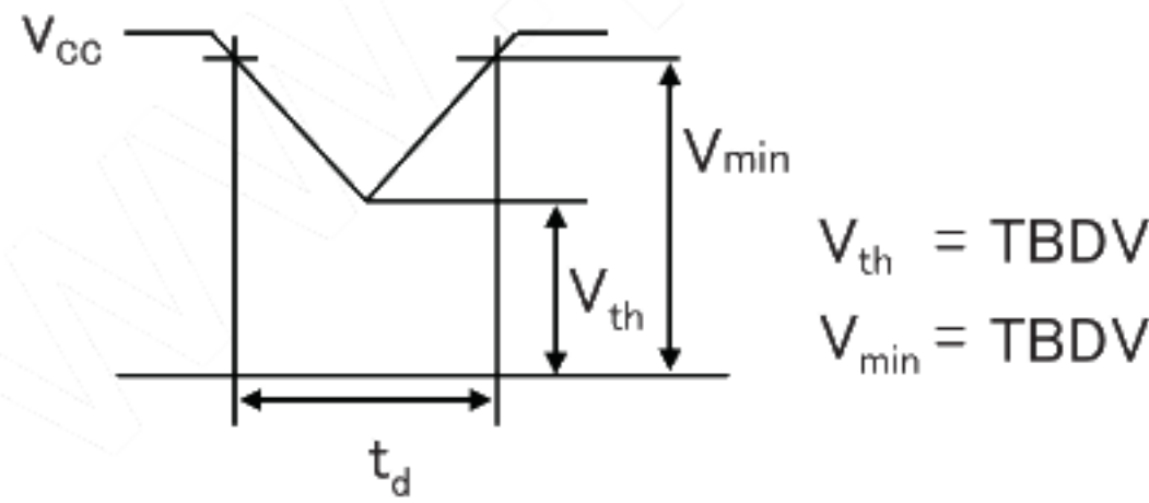
瞬時電圧降下 V CC -dip conditions
