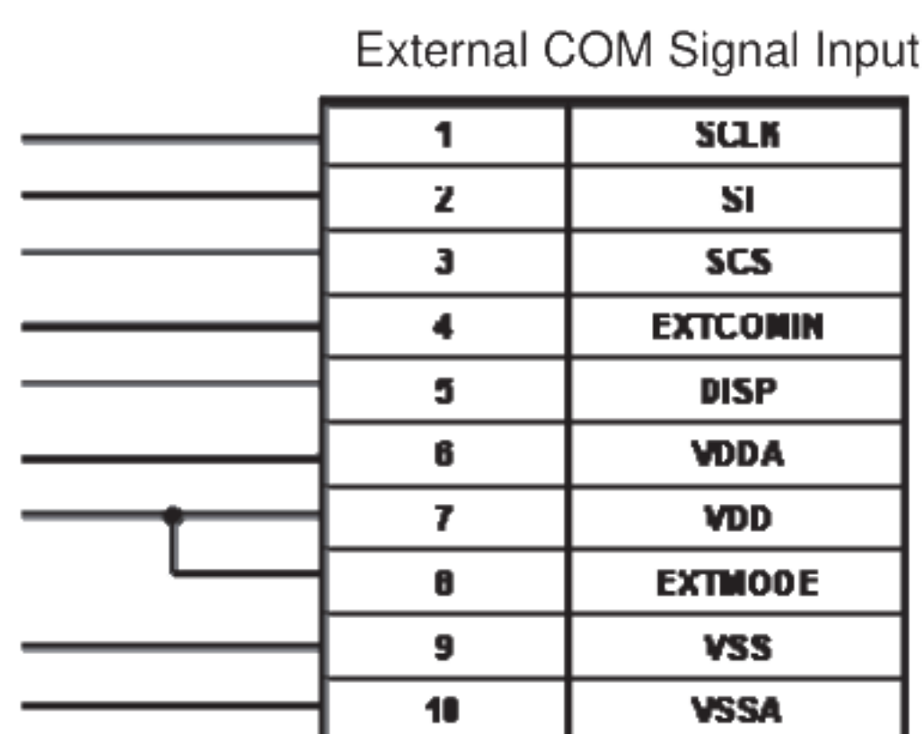
Fig 4-2 EXTMODE_Hi
