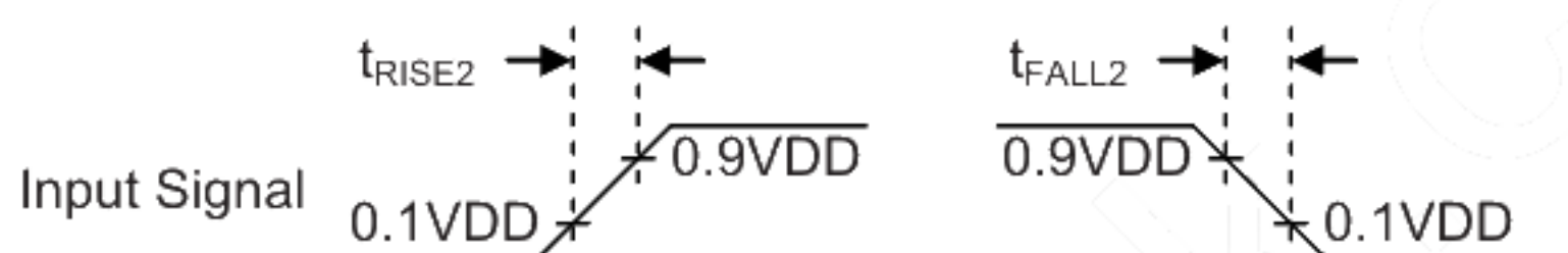
【Fig 7-2 Input Signal Rising/Falling Timing】
