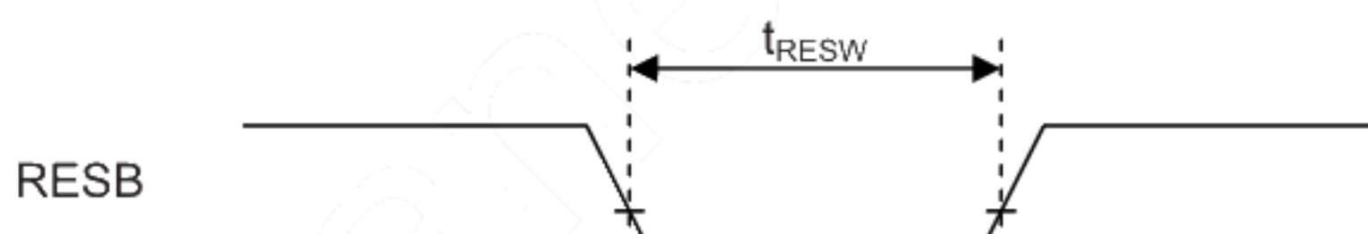
【Fig 7-3 Reset Timing Signal】
