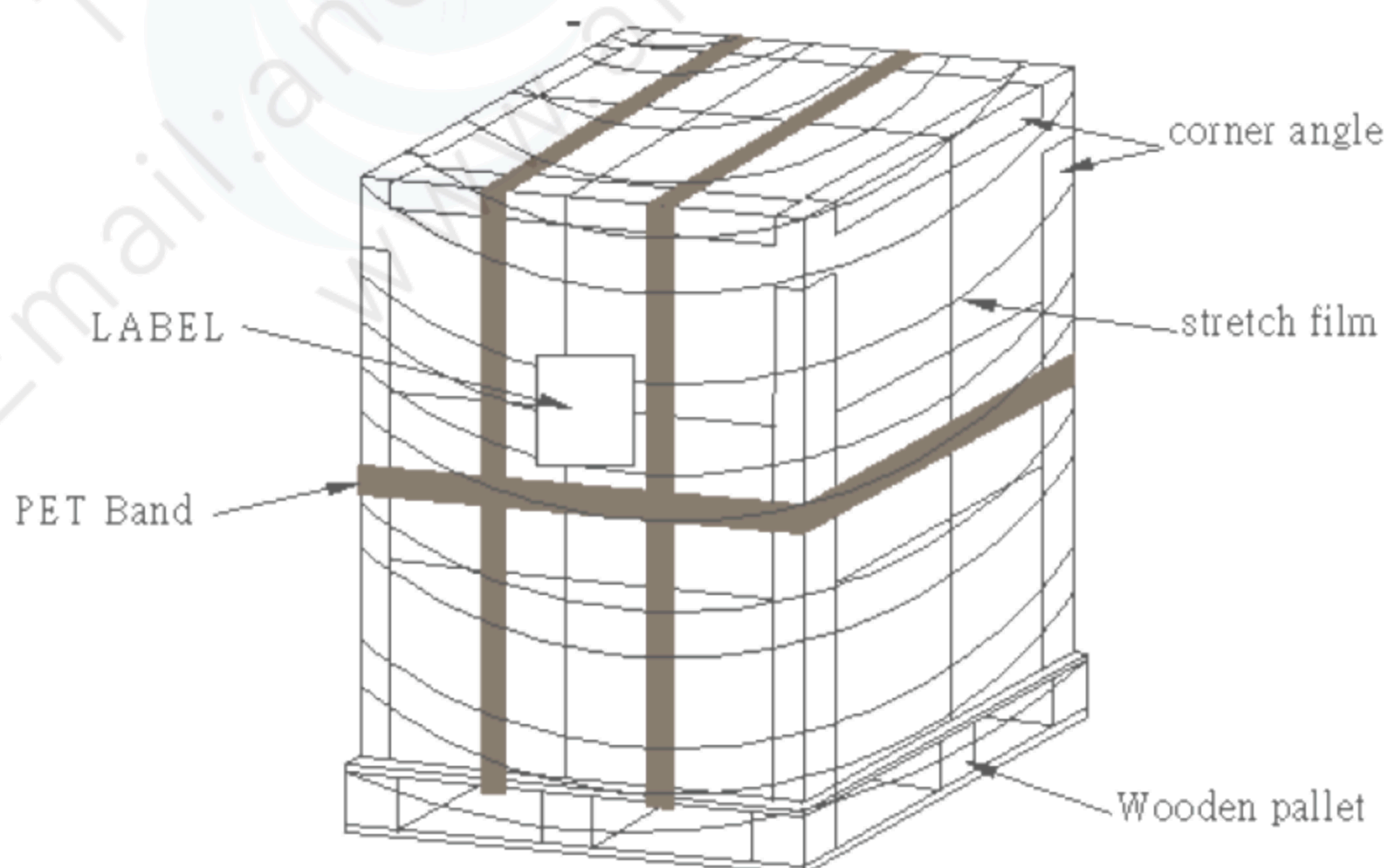
單層 pallet 打棧示意圖
