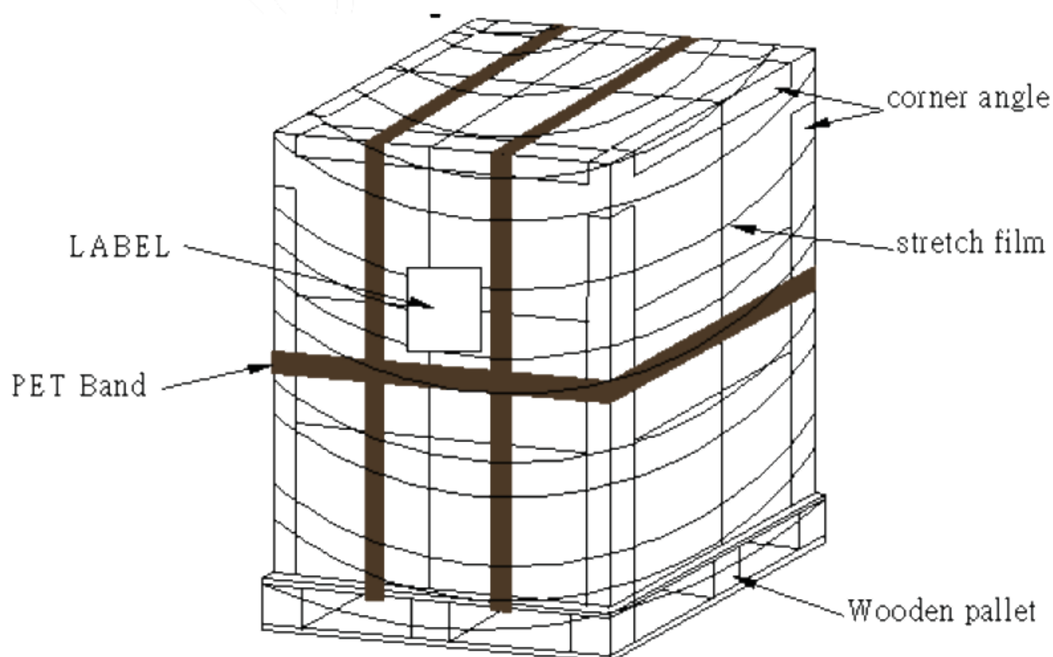
單層 pallet 打棧示意圖
