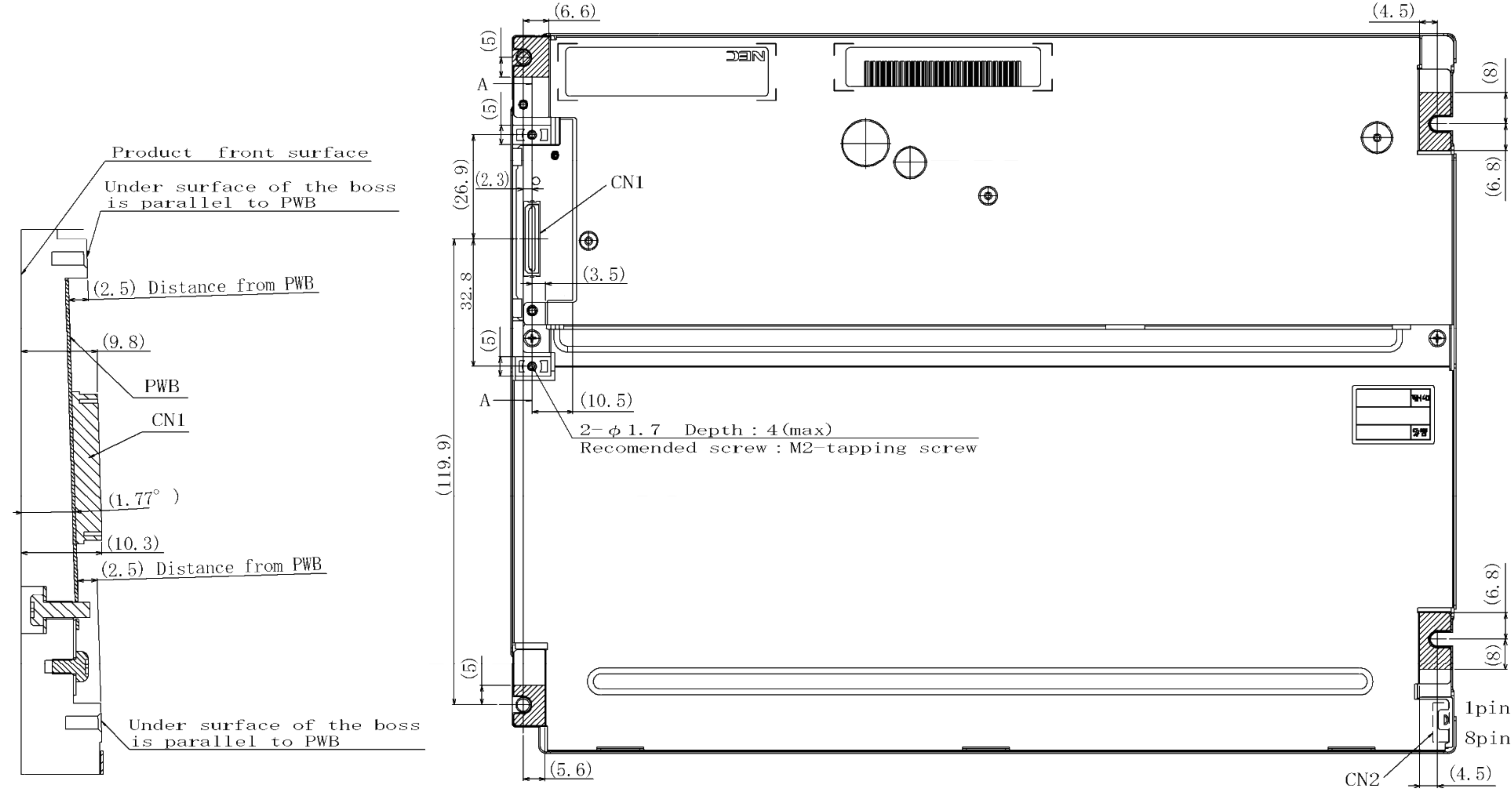
Sec. A-A
