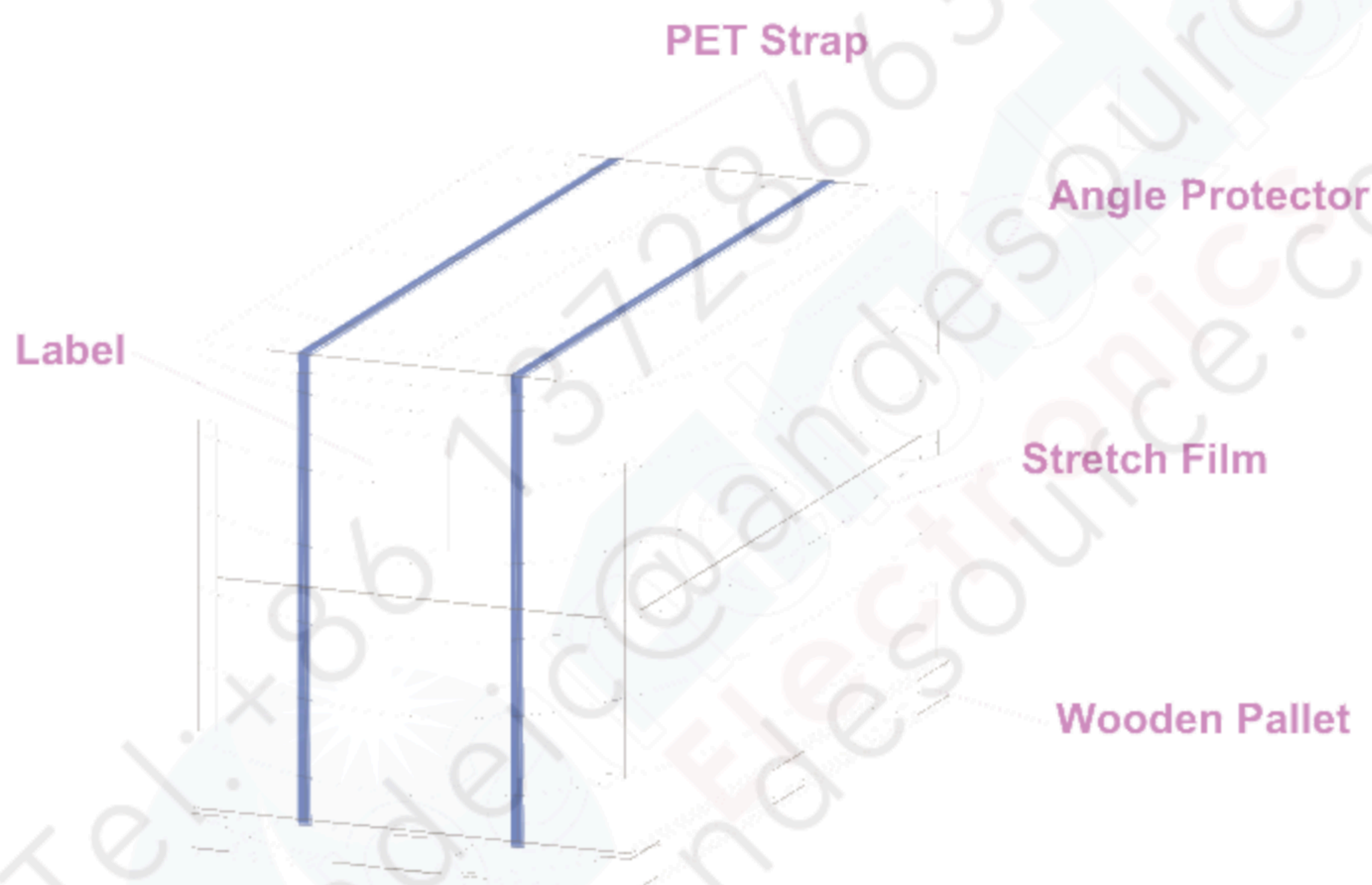
單棧 pallet 打棧示意圖
